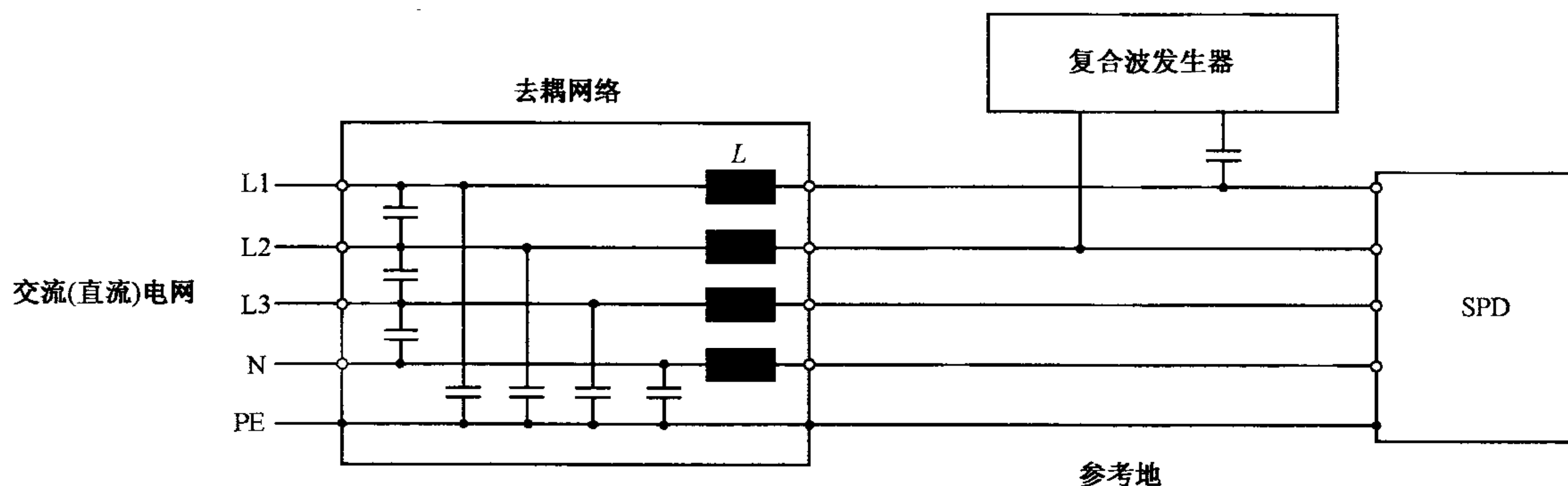
图 2 用于三相电源去耦网络的示例
