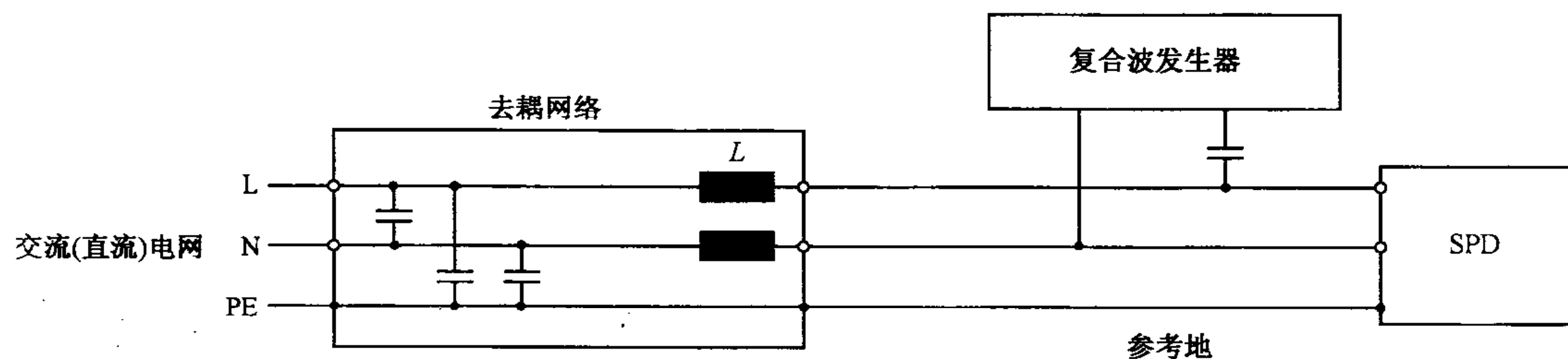
图 1 用于单相电源去耦网络的示例
