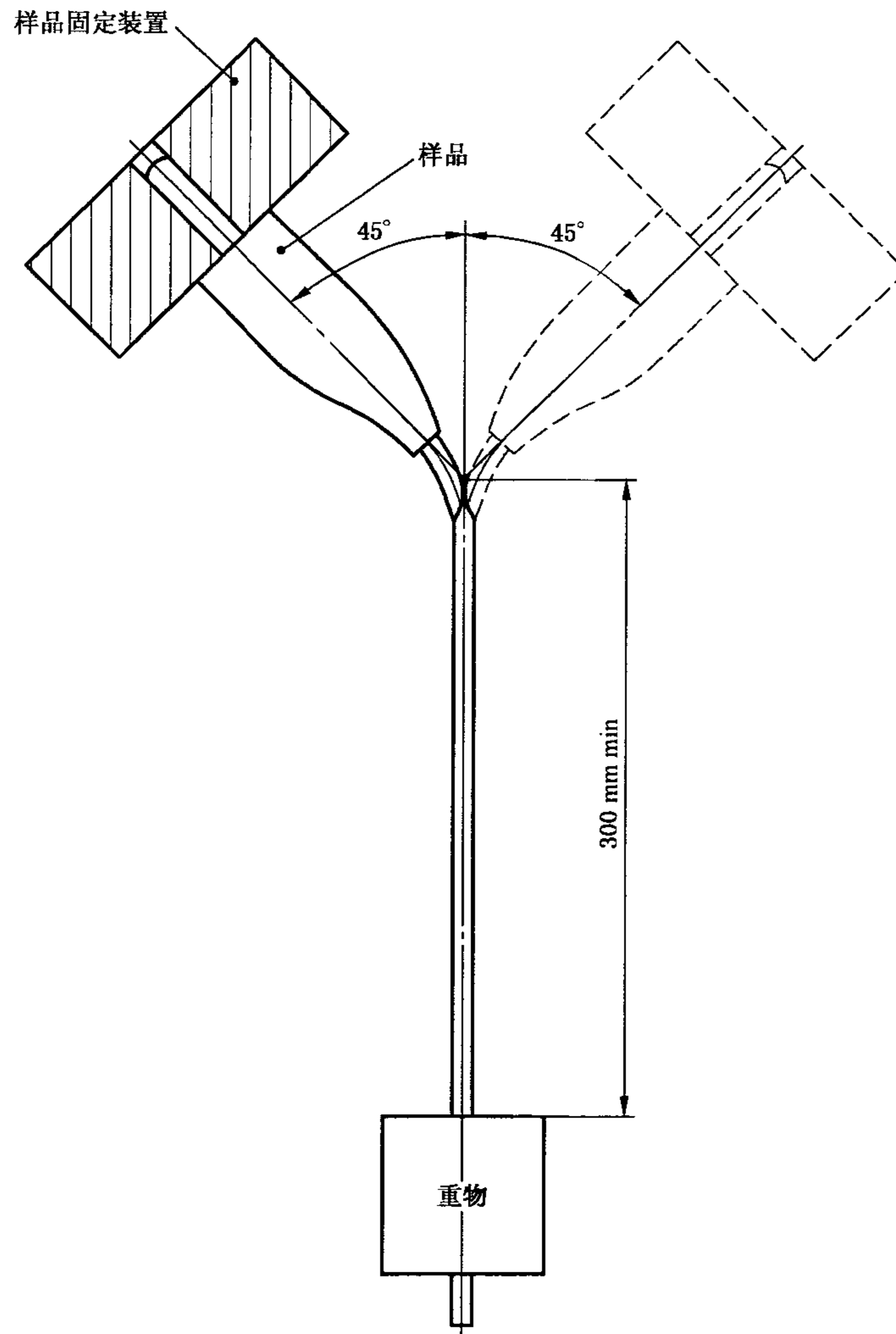
图 10 弯曲试验装置
