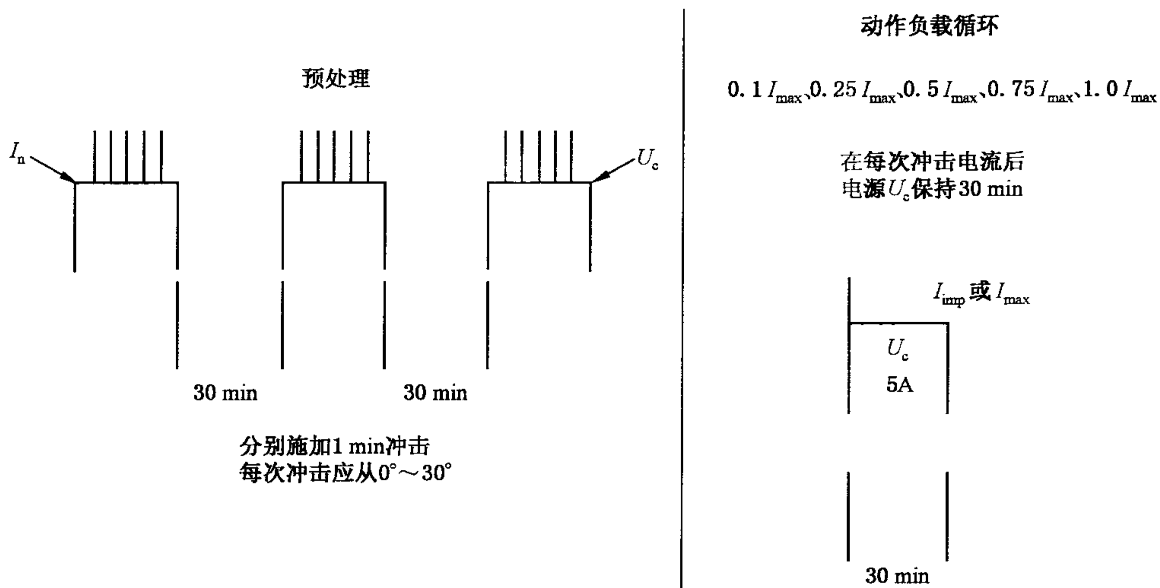
图 6 预处理和动作负载循环试验程序
