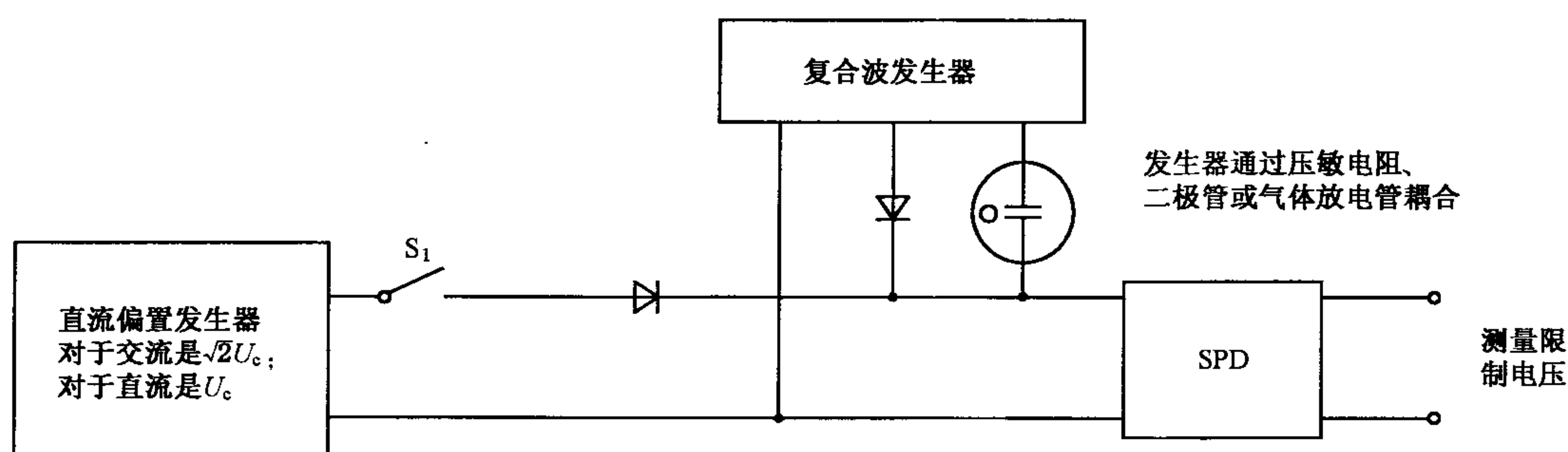
图 4 测量限制电压的替代试验
