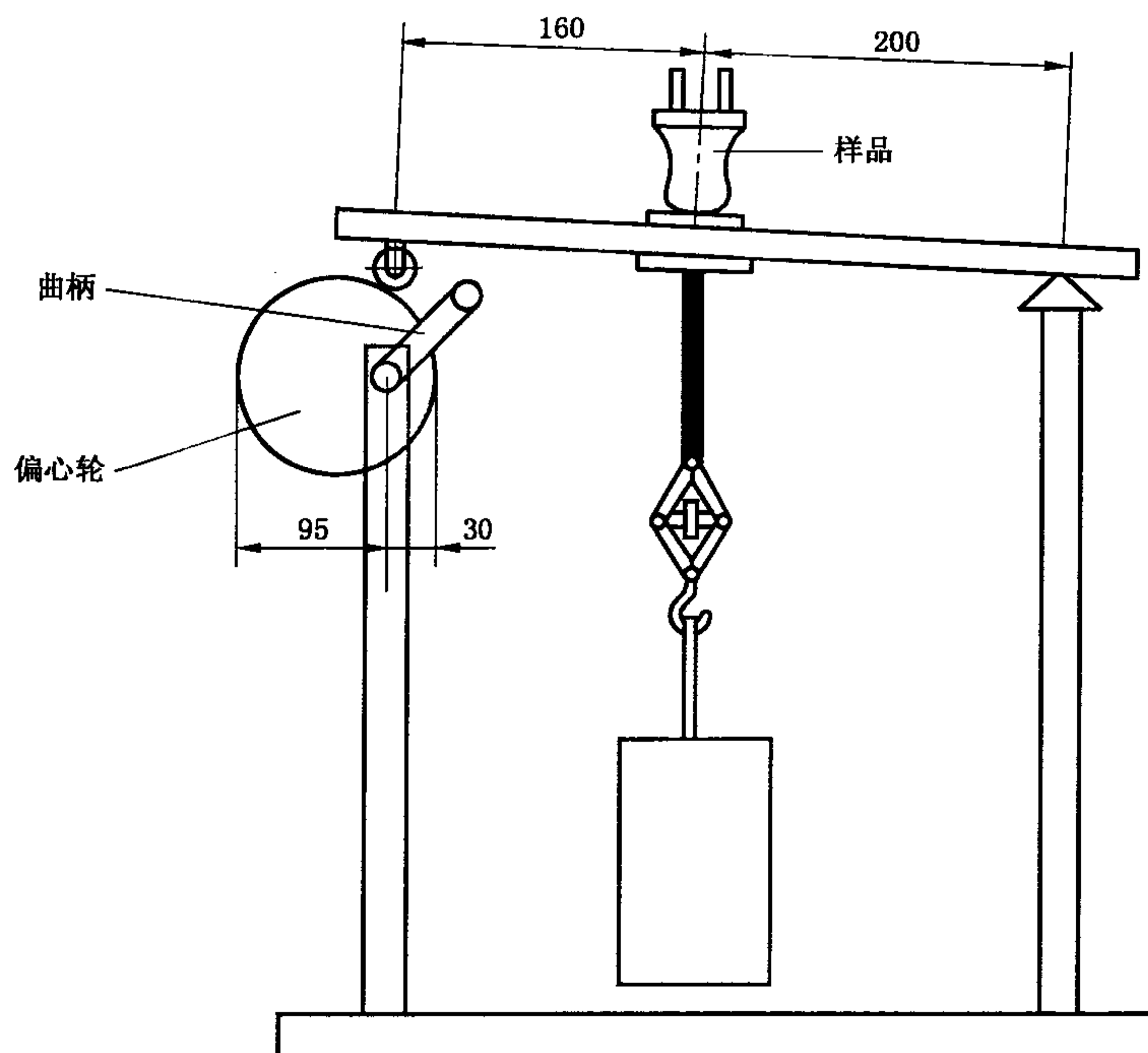
图 9 电缆保持力的试验装置
