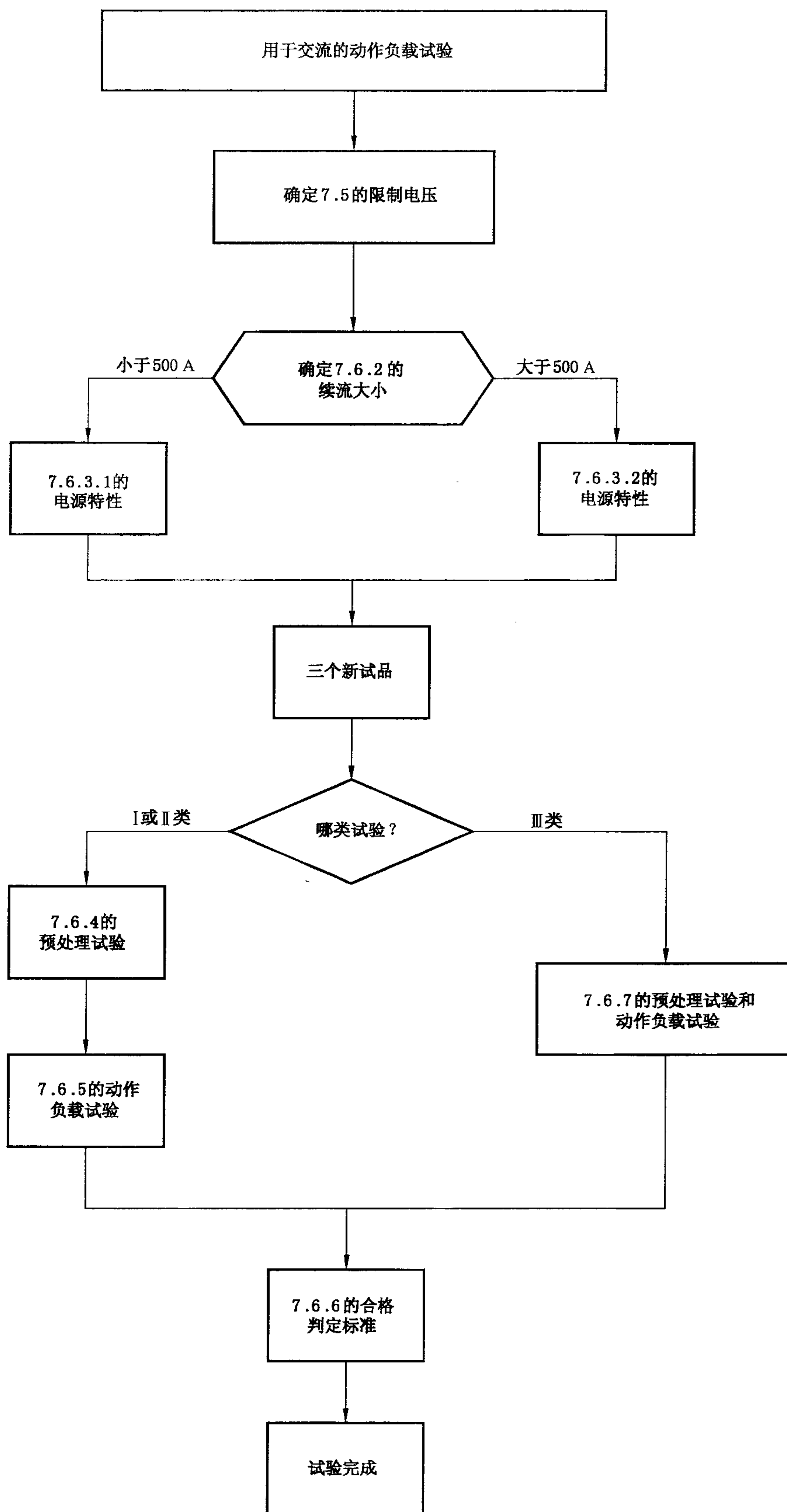
图5 动作负载试验的流程图
