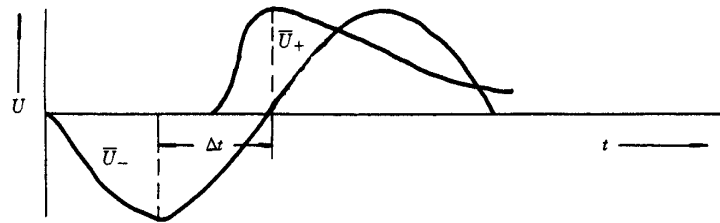
b2 一个工频电压波和一个冲击电压的联合试验
