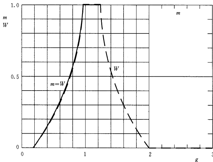
图 3 空气密度校正指数 m 值和湿度校正指数 W 与参数 g 的关系曲线
